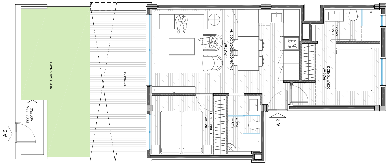
VIVIENDA A2. E 1: 100
