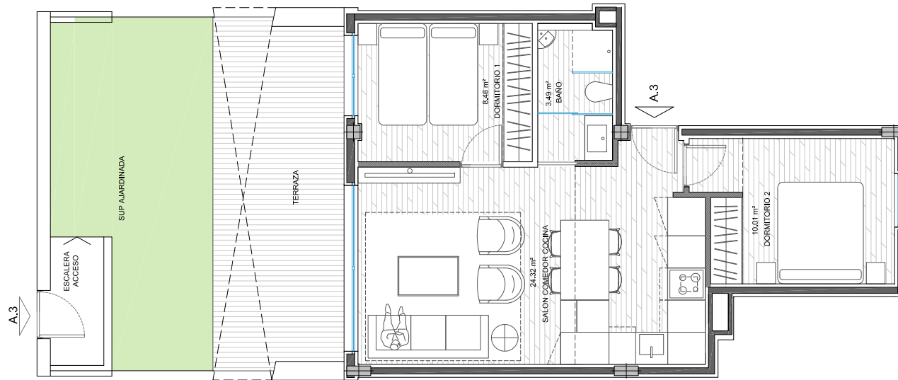
VIVIENDA A.3. E 1: 100
