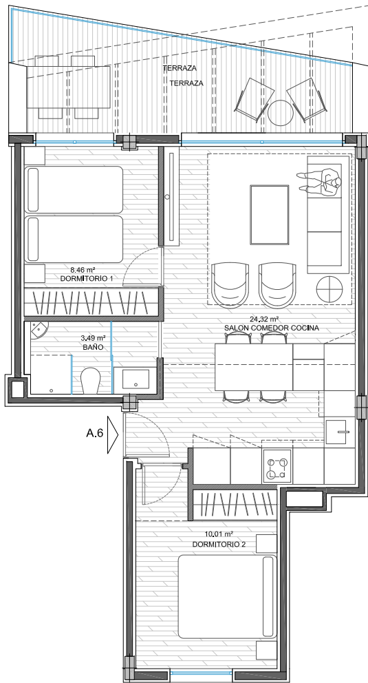
VIVIENDA A6. PLANTA PRIMERA. E 1: 100
