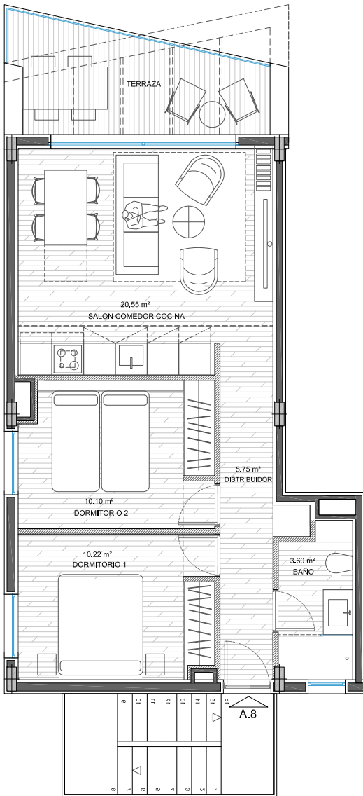
VIVIENDA A.8. PLANTA PRIMERA. E 1: 100
