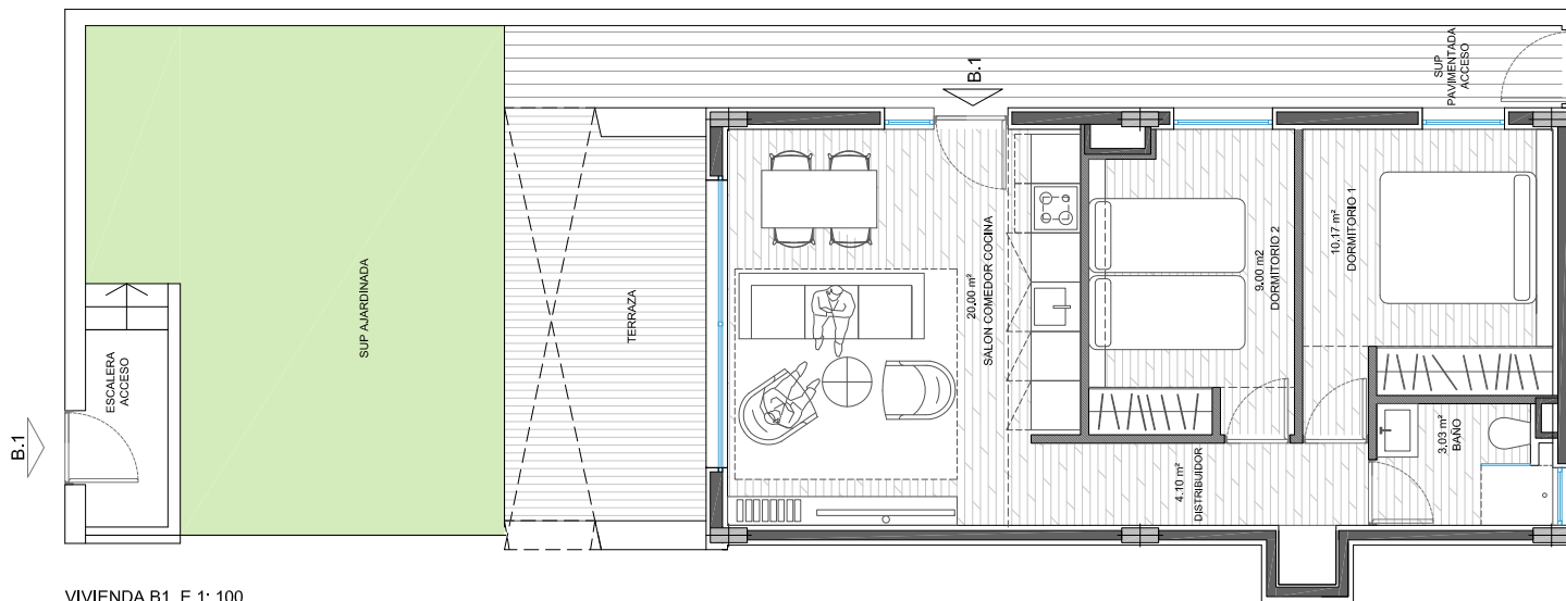
VIVIENDA B1. E 1: 100
