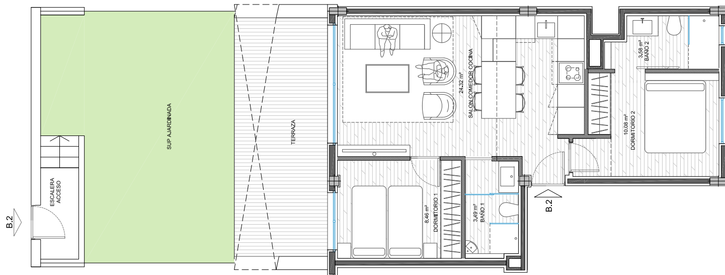
VIVIENDA B2. E 1: 100
