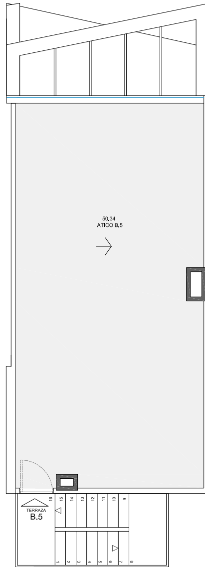
VIVIENDA B.5. PLANTA CUBIERTA. E 1: 100
