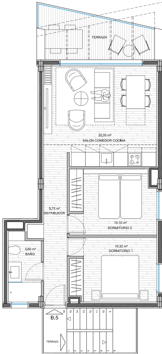
VIVIENDA B.5. PLANTA PRIMERA. E 1: 100
