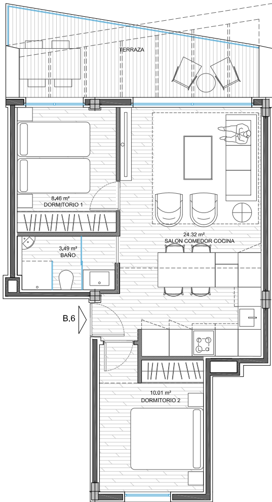
VIVIENDA B6. PLANTA PRIMERA. E 1: 100
