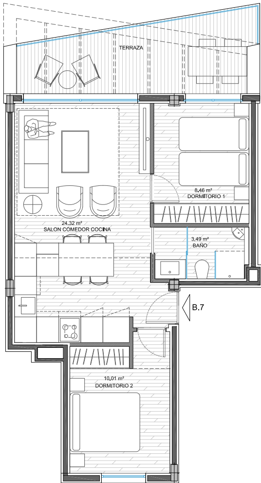
VIVIENDA B7, PLANTA PRIMERA, E 1: 100
