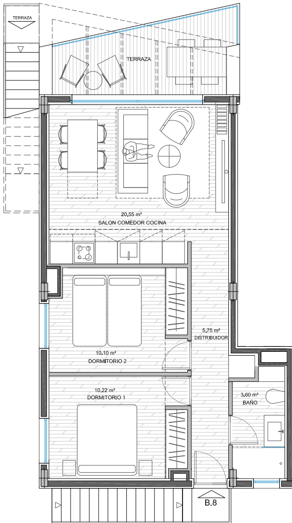
VIVIENDA B8. PLANTA PRIMERA. E 1: 100
