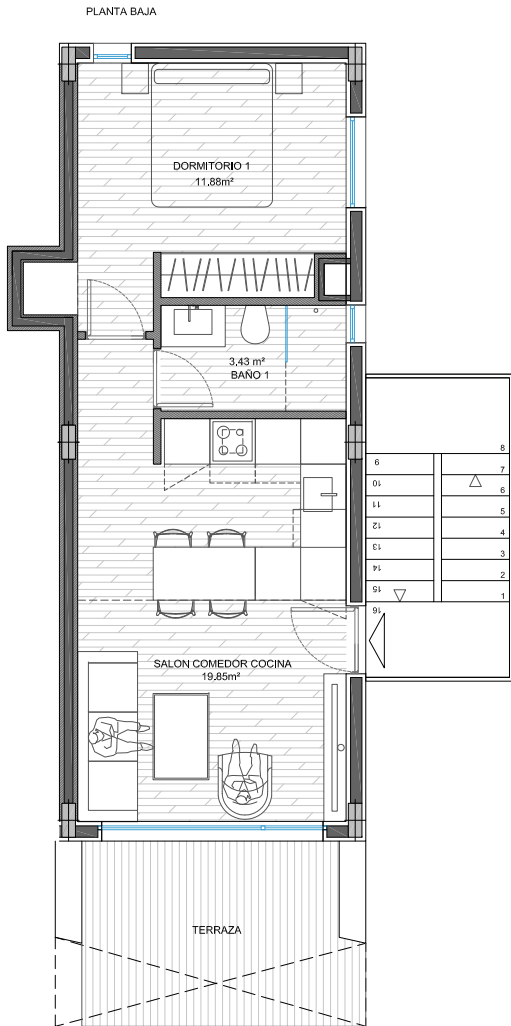
VIVIENDA C5. PLANTA PRIMERA. E 1: 100
