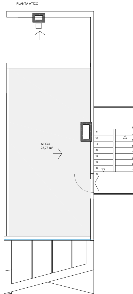
VIVIENDA C5. PLANTA CUBIERTA. E 1: 100
