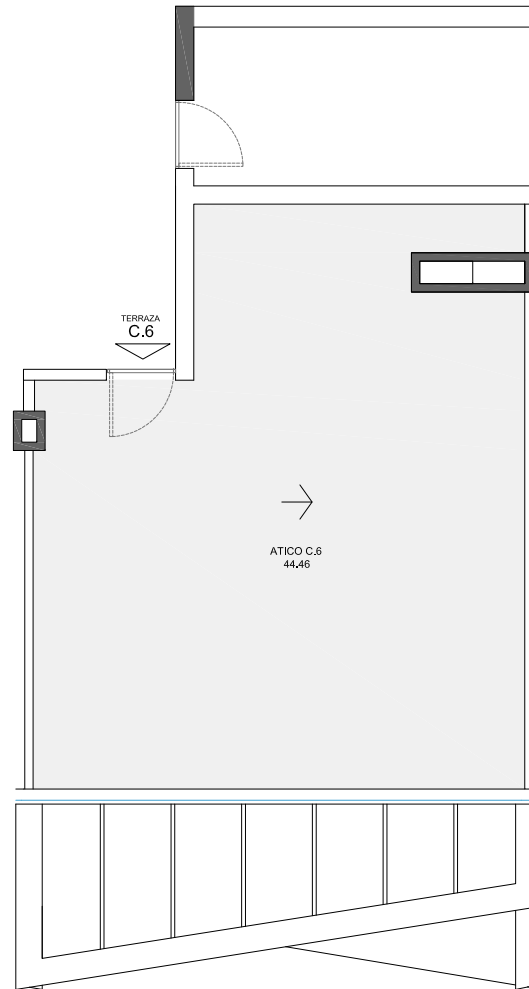
VIVIENDA C6. PLANTA CUBIERTA. E 1: 100
