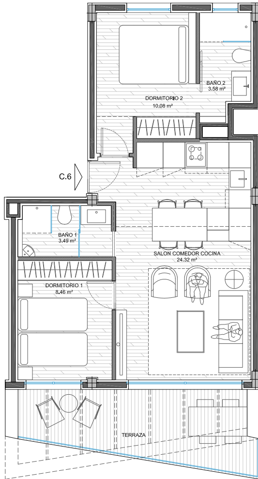
VIVIENDA C6. PLANTA PRIMERA. E 1: 100
