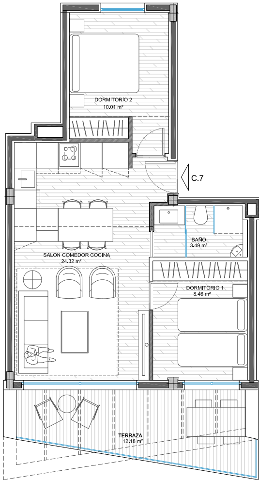
VIVIENDA C7. PLANTA PRIMERA. E 1: 100
