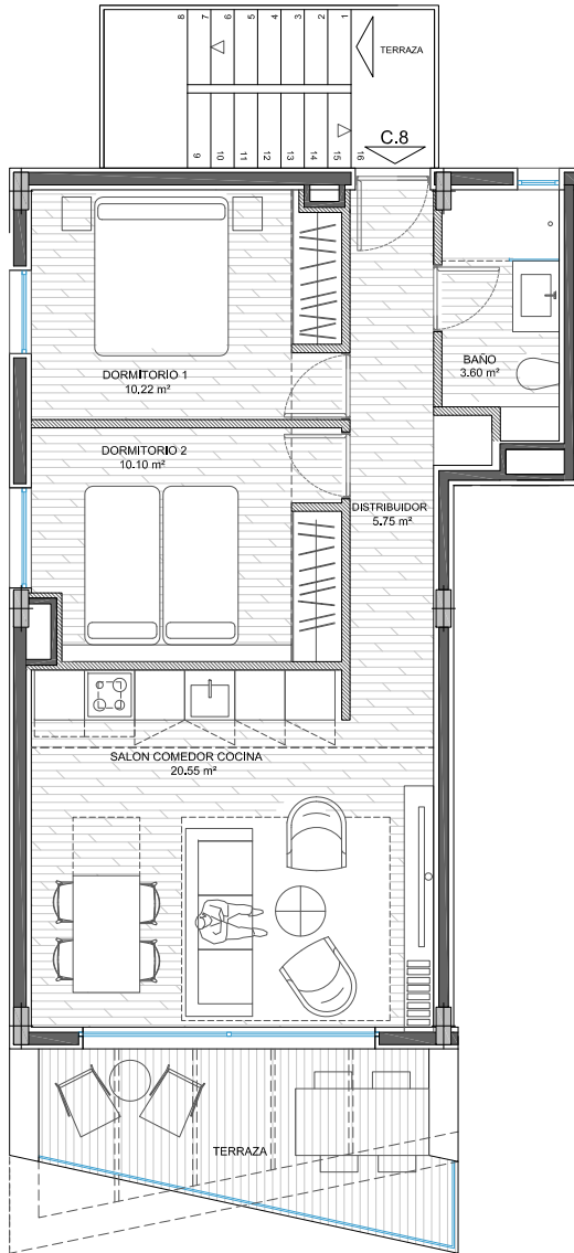
VIVIENDA C8. PLANTA PRIMERA. E 1: 100
