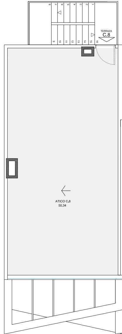
VIVIENDA C8. PLANTA CUBIERTA. E 1: 100
