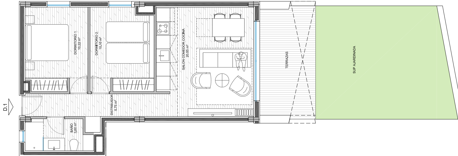
VIVIENDA D1. E 1: 100
