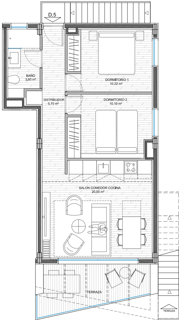
VIVIENDA D5. PLANTA PRIMERA. E 1: 100
