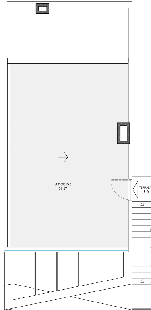
VIVIENDA D5. PLANTA CUBIERTA. E 1: 100
