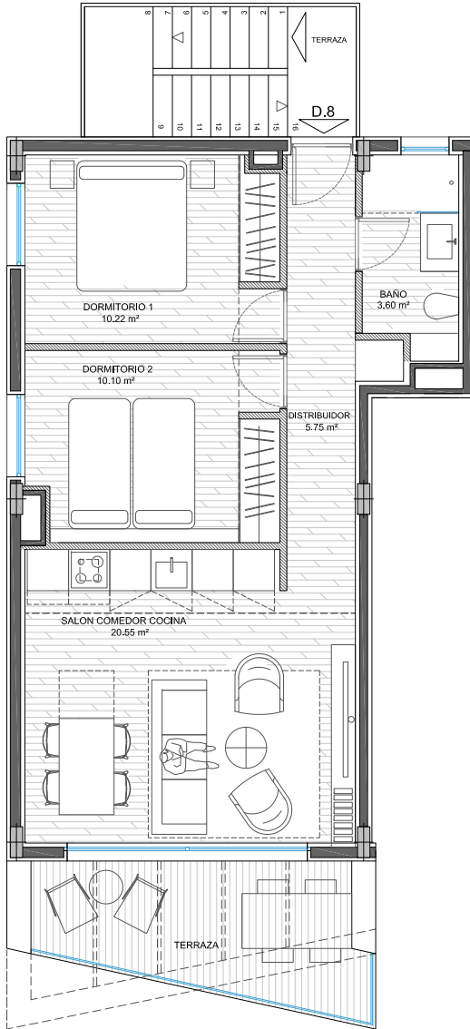
VIVIENDA D8. PLANTA PRIMERA. E 1: 100
