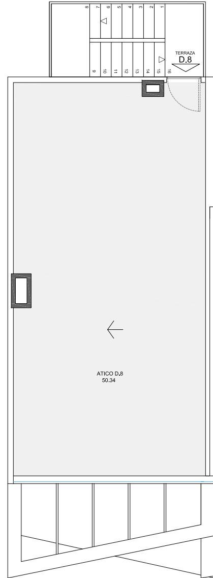
VIVIENDA D8. PLANTA CUBIERTA. E 1: 100
